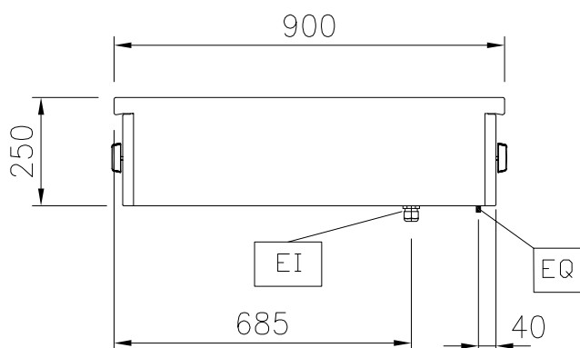
Zij aanzicht
