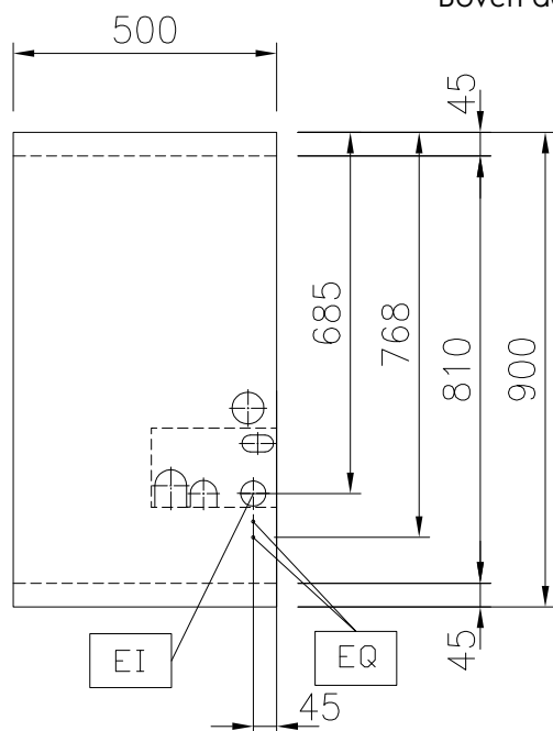
Boven aanzicht
